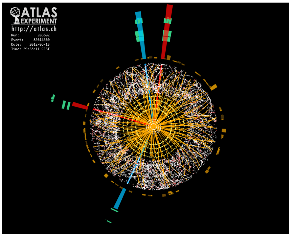
Figura 1. Candidato a Higgs decaindo em 4 elétrons observado pela experiência ATLAS em 2012.
