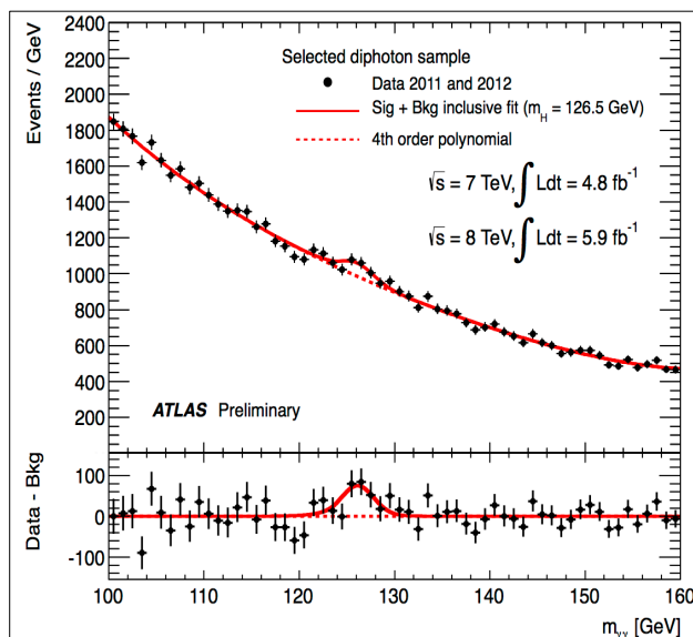
Figura 3. Distribuição da Massa para o canal de dois fótons.
