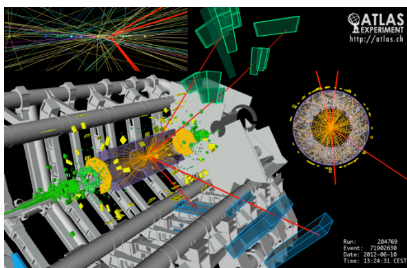
Figura 2. Candidato a Higgs decaindo em quatro múons observado pela experiência ATLAS em 2012.
