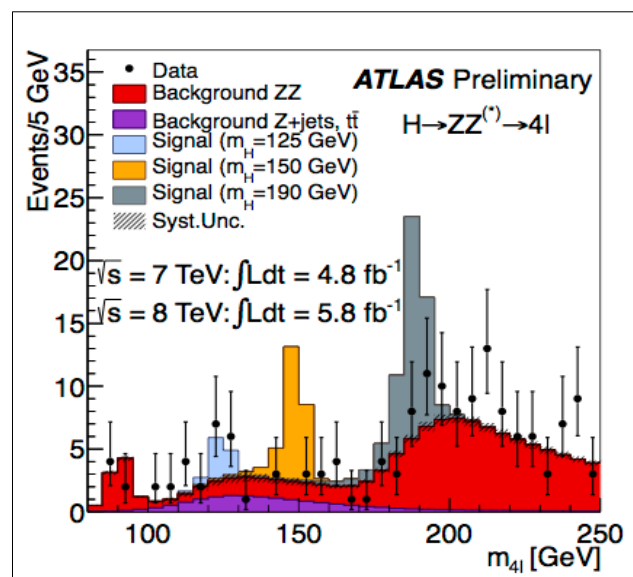
Figura 3. Distribuição da Massa para o canal de quatro léptons.
